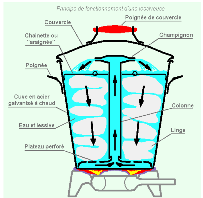
Fonctionnement d'une lessiveuse
